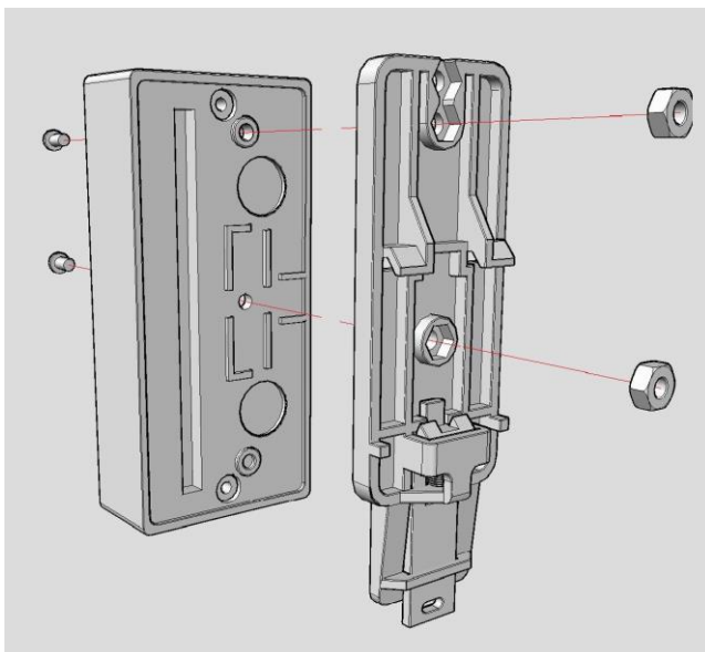
Figure 22: DIN rail clip fitting detail – Specify DIN Rail Mounting Kit P/N 290407157
