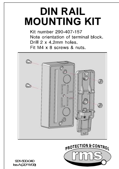
Figure 22: DIN rail clip fitting detail – Specify DIN Rail Mounting Kit P/N 290407157
